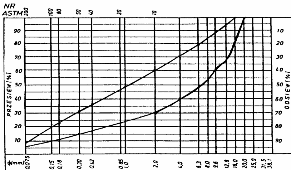
Rys. 1. Krzywe graniczne uziarnienia mieszanki mineralnej 0+20 mm do warstwy ścieralnej z betonu asfaltowego dla KR 1-2
