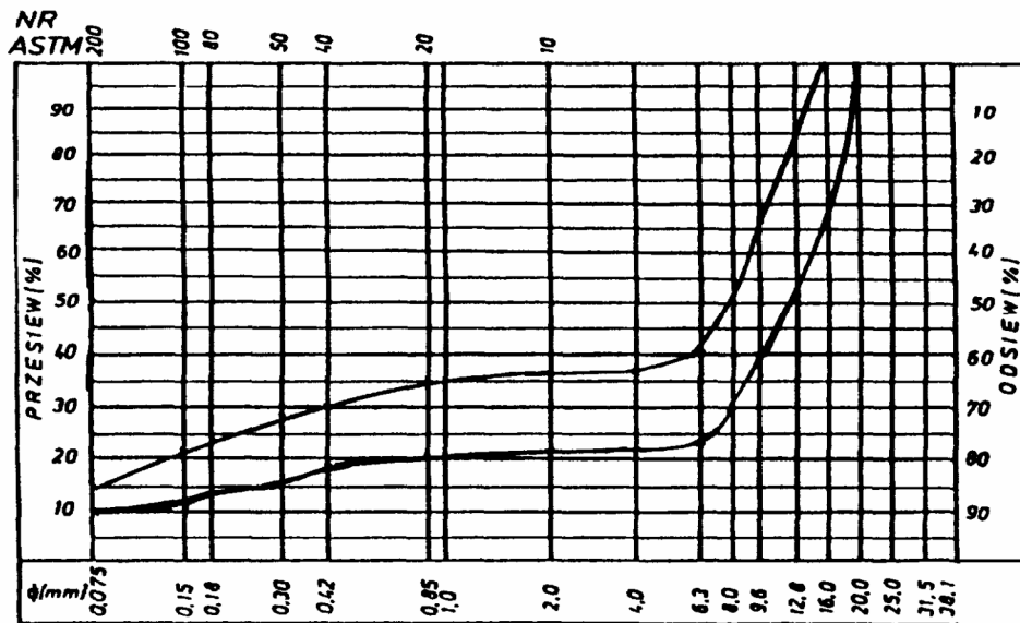
Rys. 4. Krzywe graniczne uziarnienia mieszanki mineralnej 0+20 mm do warstwy ściernalnej z betonu asfaltowego dla KR 3-6
